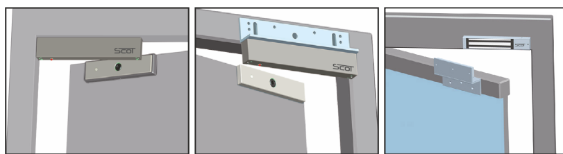
Montaż standardowy / z uchwytem BK-600I2
