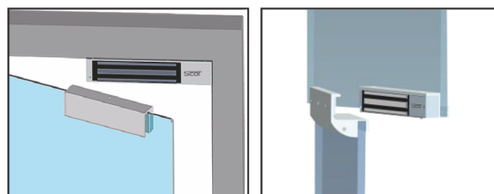
Montaż z uchwytem BK-600UL
