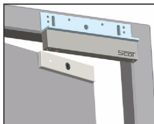
Montaż z uchwytem BK-350L, BK-350LC
