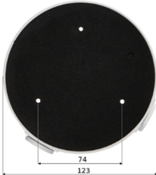
Widok od strony mocowania do ściany:
