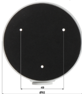
Widok od strony mocowania do ściany:
