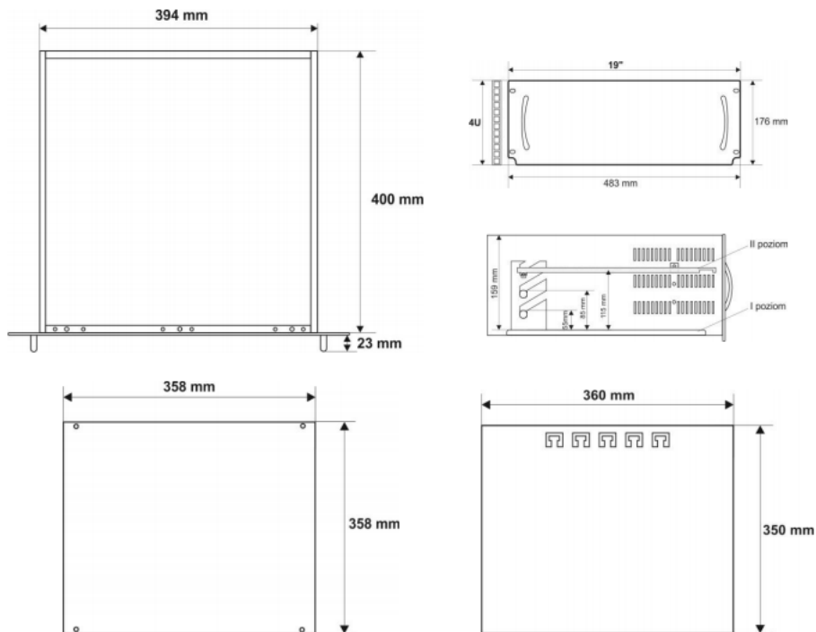
Wymiary blachy montażowej i blachy uchylnej
