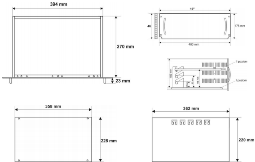
Wymiary blachy montażowej i blachy uchylnej
