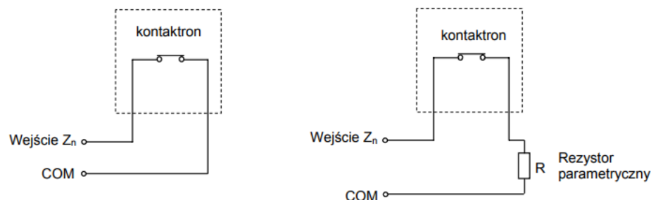
Powszechnie stosowany sposób podłączenia czujki magnetycznej
