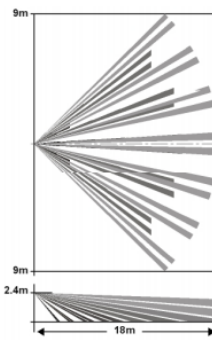
Rys. 2 – Soczewka kurtynowa dalekiego zasięgu – OPCJA
