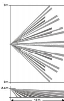
Rys. 2 – Soczewka kurtynowa dalekiego zasięgu – OPCJA
